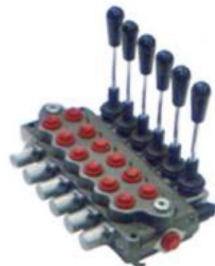
Distribuidor hidráulico (6 palancas)
